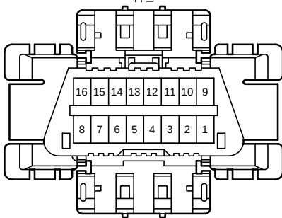
90980-11665
