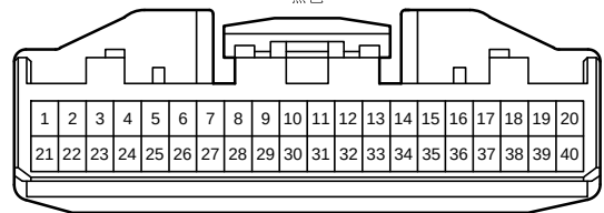
90980-12557
