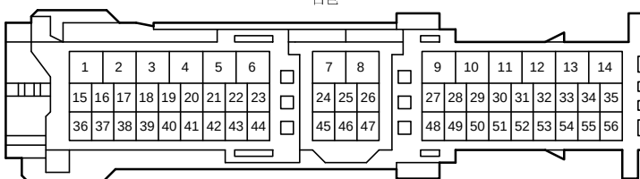
90980-12A15
